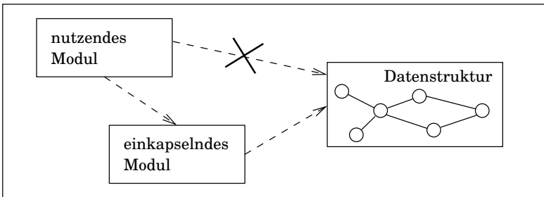
Abbildung 1: Datenkapselung im Programm
