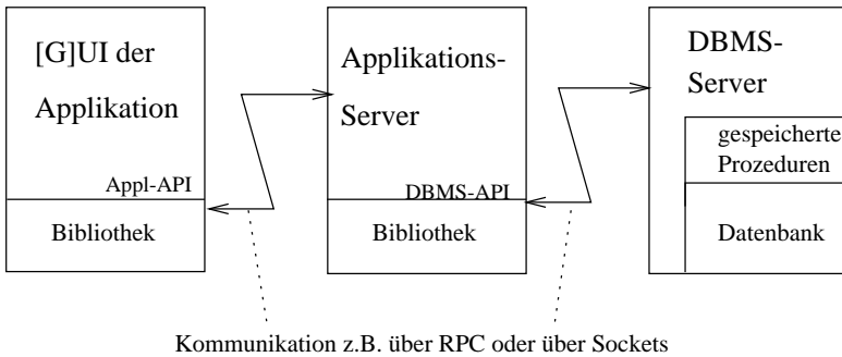
Abbildung 2: Prozeßarchitektur von Informationssystemen mit gespeicherten Prozeduren
