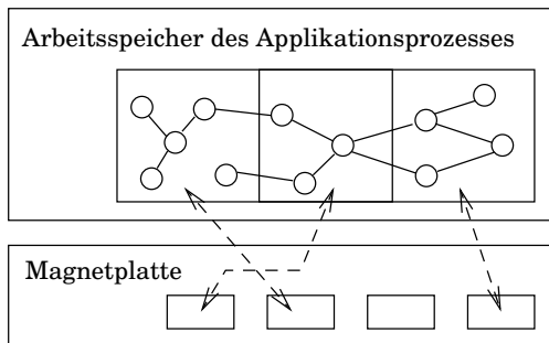
Abbildung 3: Seitenorientierte Verfahren
